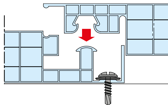
Particolare di aggancio lastre
