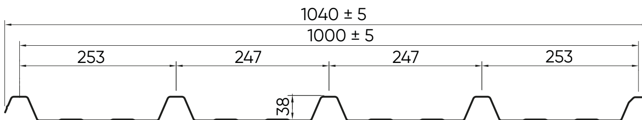
SILEX Spessore 1 mm
