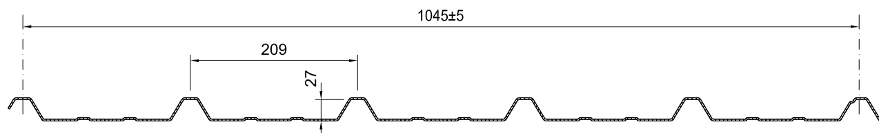
ISOCOPRE / PROFILCASTELLO 6 greche Spessore 2,5 mm
