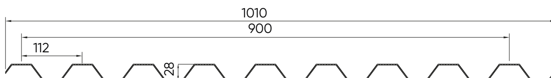
GRECA ALUBEL 28/112 9 greche Spessore 2,5 mm
