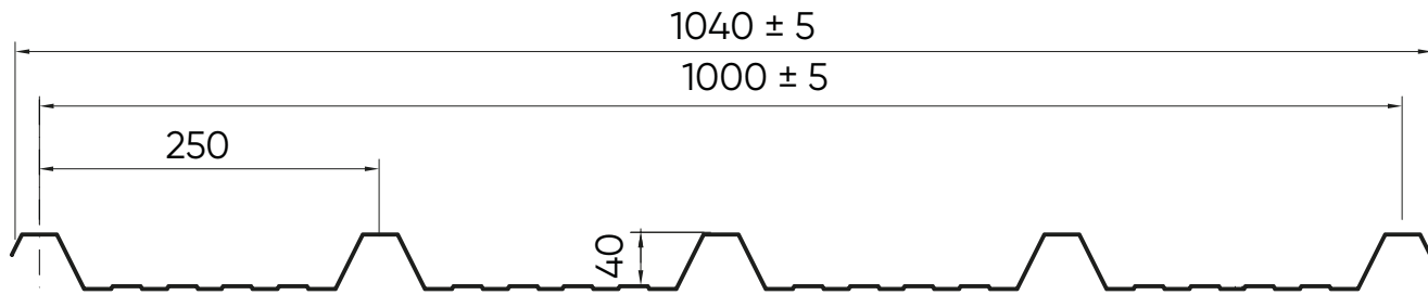
ISOCOPRE/PROFILCASTELLO 6 greche Spessore 1 mm
