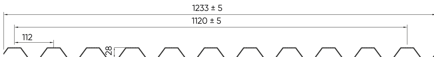
GRECA ALUBEL 28/112 10 greche Spessore 2,5 mm
