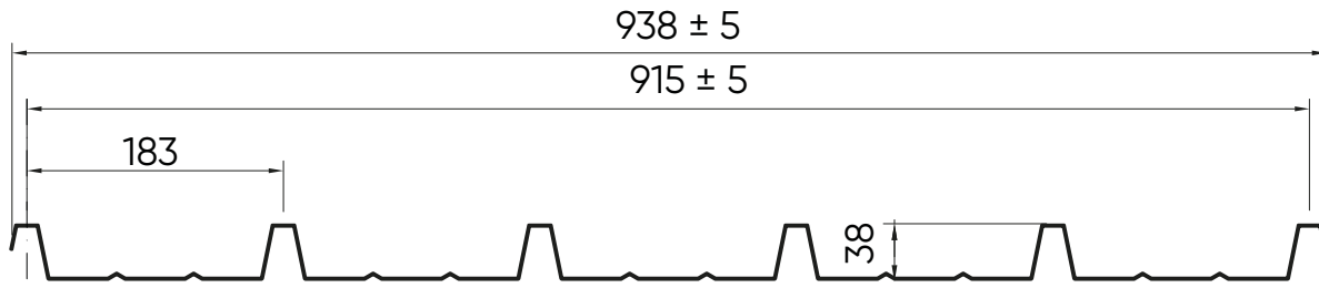
EUROFIRE Spessore 1 mm
