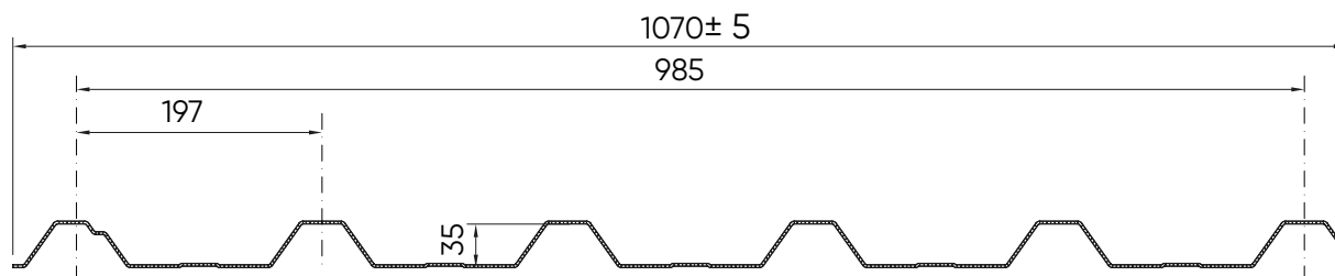
SILMA 6 greche Spessore 2,5 mm
