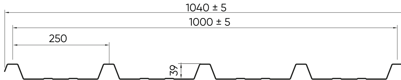
ISOLPACK 5 greche Spessore 1 mm
