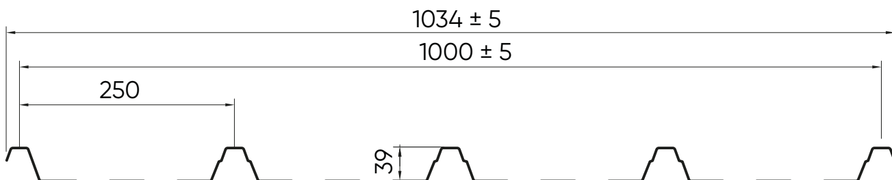
Italpanelli 5 greche Spessore 1 mm
