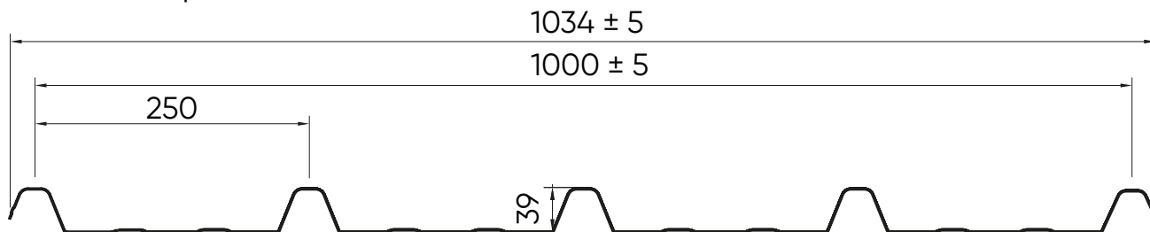
EUROFIRE Spessore 1 mm
