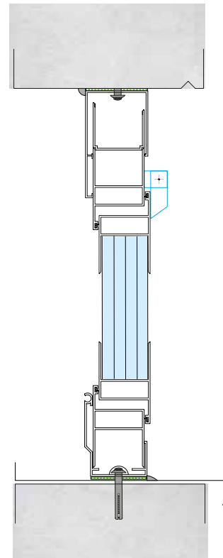
Sezione apribile su shed a parete Profili a taglio termico
