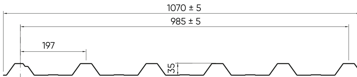
SILMA 6 Spessore 1 mm
