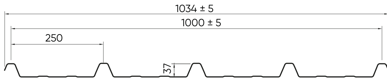
LATTONEDIL 5 greche Spessore 1 mm
