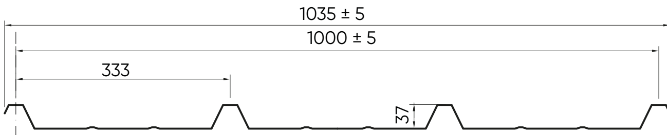
EUROCOPE Spessore 1 mm
