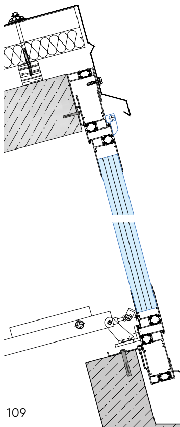
Sezione apribile su shed inclinato Profili a taglio termico
