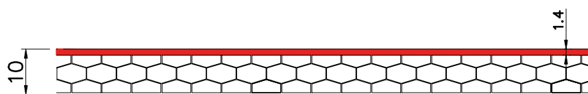
Sezione lastra Carbopiù® Alveolare Rinforzato 10 - 16 - 20 mm
