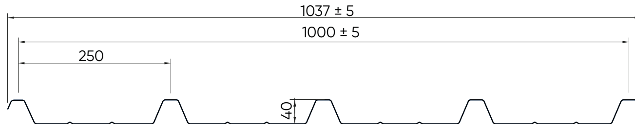
ISOPAN 5 greche Spessore 1 mm
