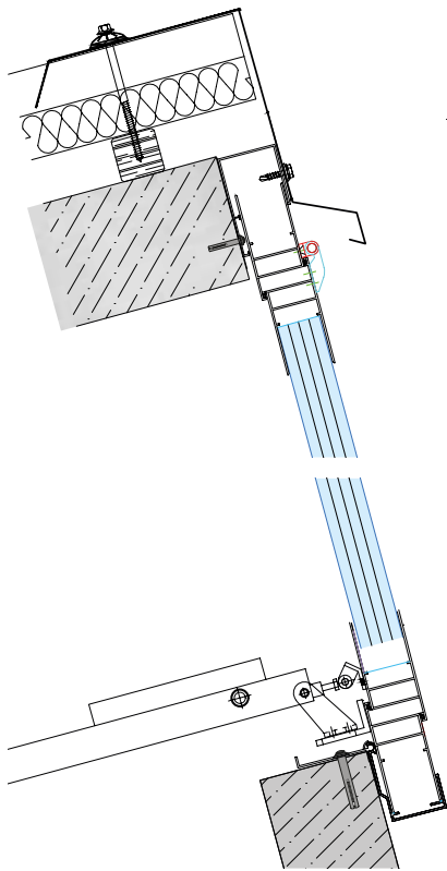
Sezione apribile su shed inclinato Profili a taglio freddo
