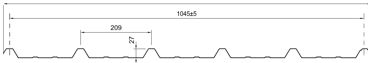
SILMA 6 Spessore 1 mm
