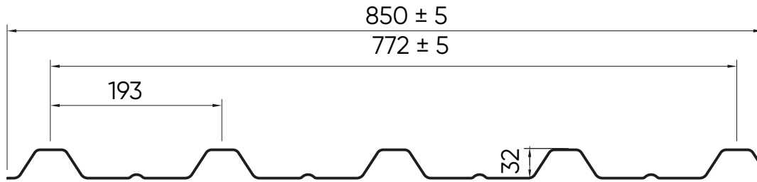
COVERIB 1000 Spessore 1 mm
