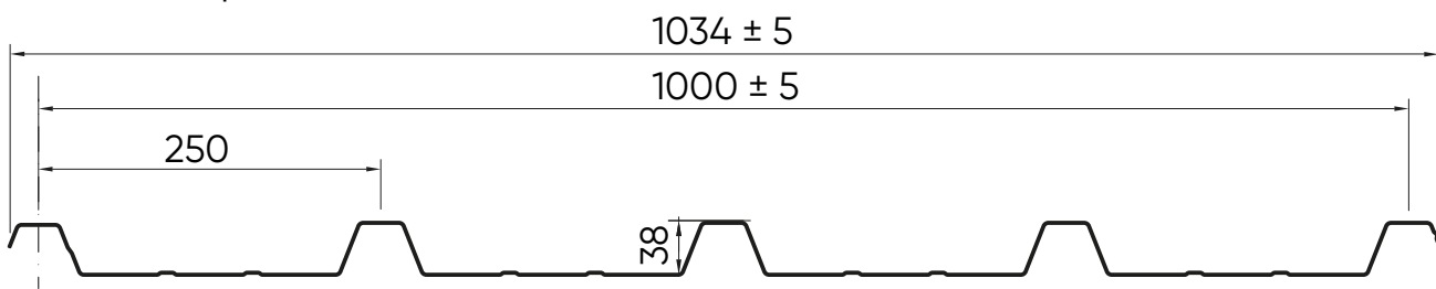
POLYPIVA Spessore 1 mm
