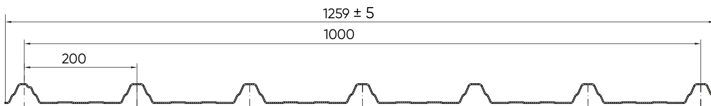
SAND 27 6 greche Spessore 2,5 mm
