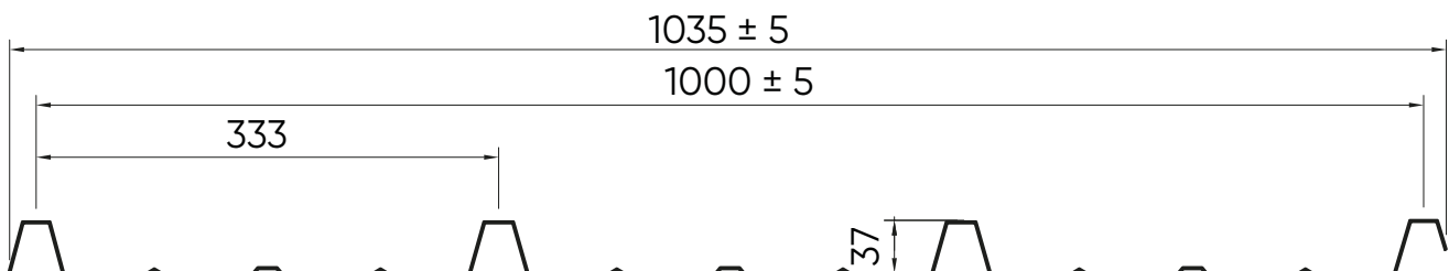
METECNO Spessore 1 mm
