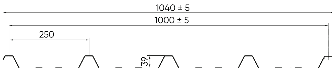
SAND 40 Spessore 1 mm
