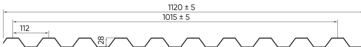
GRECA ALUBEL 28/112 10 greche Spessore 2,5 mm
