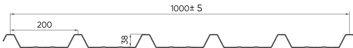
ISOCOPRE / PROFILCASTELLO 6 greche Spessore 2,5 mm
