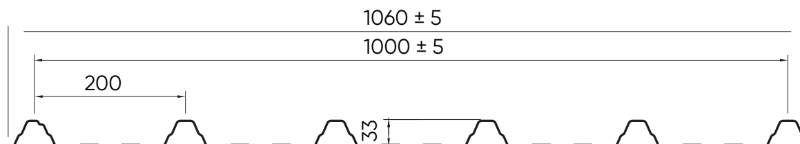
SAND 35 7 greche Spessore 1 mm
