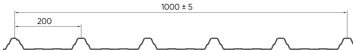
SAND 35 6 greche Spessore 2,5 mm
