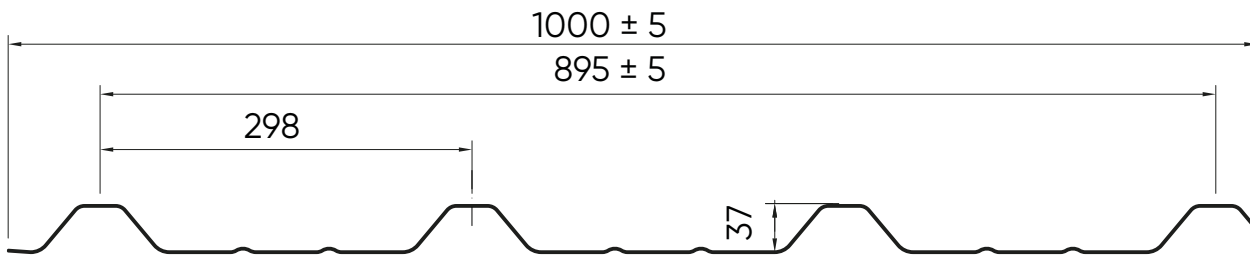
ALUBEL DACH Spessore 1 mm
